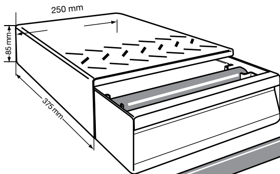
620437 BASE CON BATTIFONDI BASE WITH KNOCKBOX
