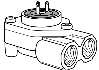
620405 1/4" UL-NSF METAL 620404 1/8" UL-NSF METAL
