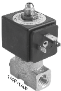
LUCIFER 0-10 bar 632018/22 V220/50/60 632018/11 V110/60 632018/24 V24/50/60
