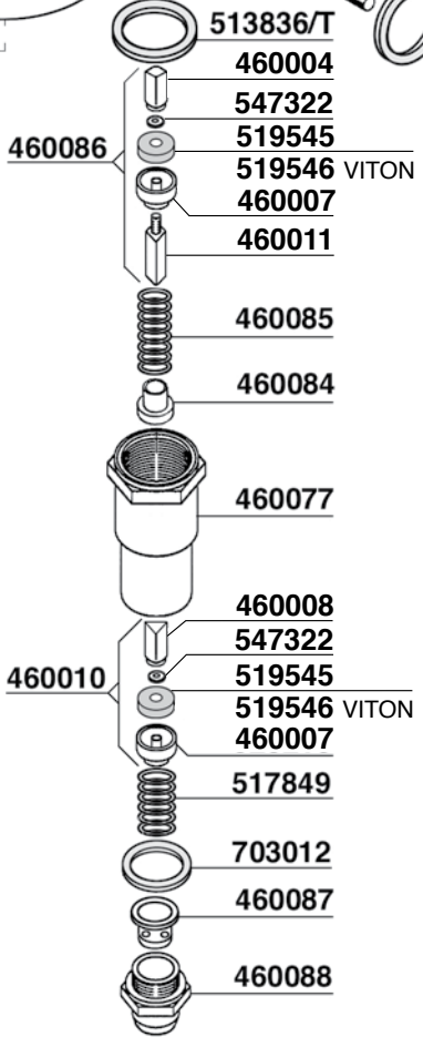
DOCCETTA DOPPIA DOUBLE SHOWER
