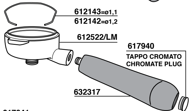
617941 TAPPO CROMATO BLU CHROMATE PLUG BLUE
