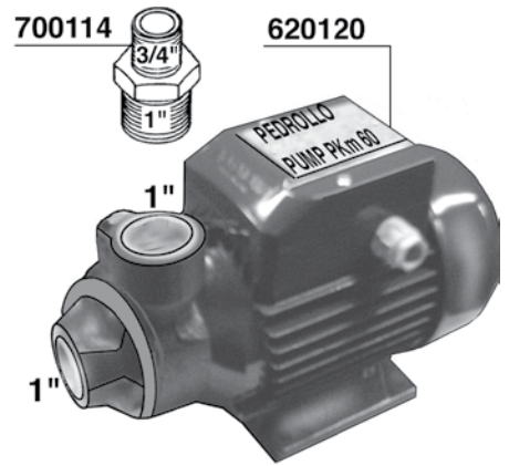
POMPA AUSILIARIA RISCIAQUO RINSE BOSTER PUMP l/min. 5 ÷ 40 H 5 ÷ 38 mt HP 0,5 V220/230
