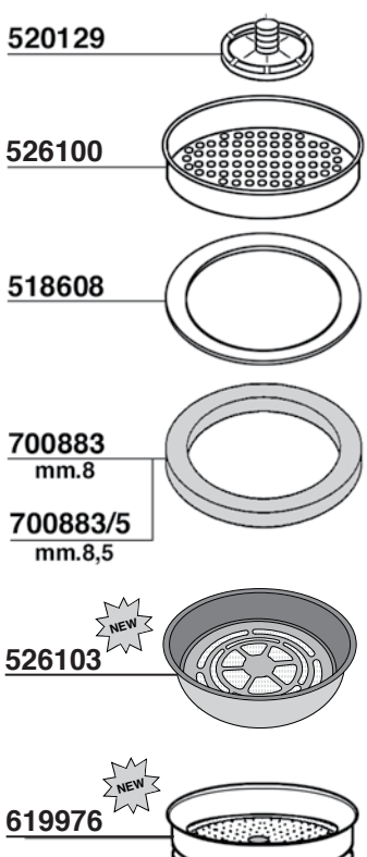
DOCGETTA DOPPIA DOUBLE SHOWER
