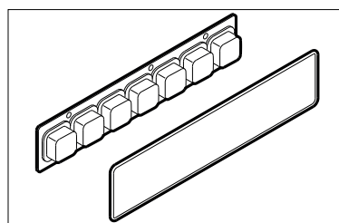
707138 SABRINA ASSIEME PULSANTIERA TOUCHPAD ASSEMBLY
