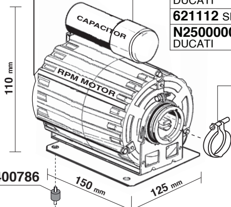
MOTORE PICCOLO - SMALL MOTOR
