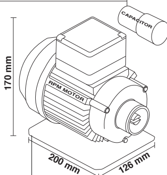
700095 V220/230-240 W150 HP0,4
